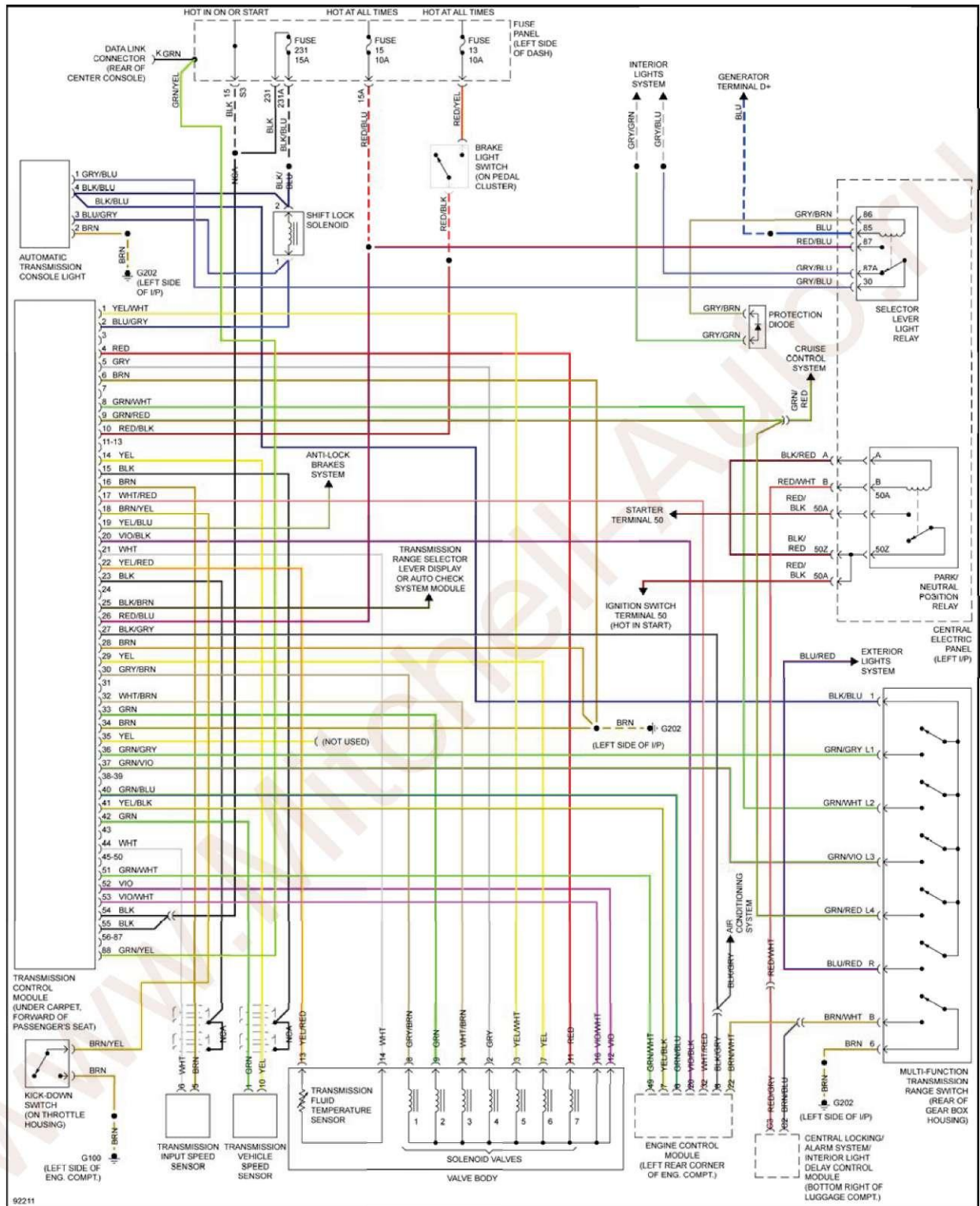
Fig. 37: A/T Circuit
