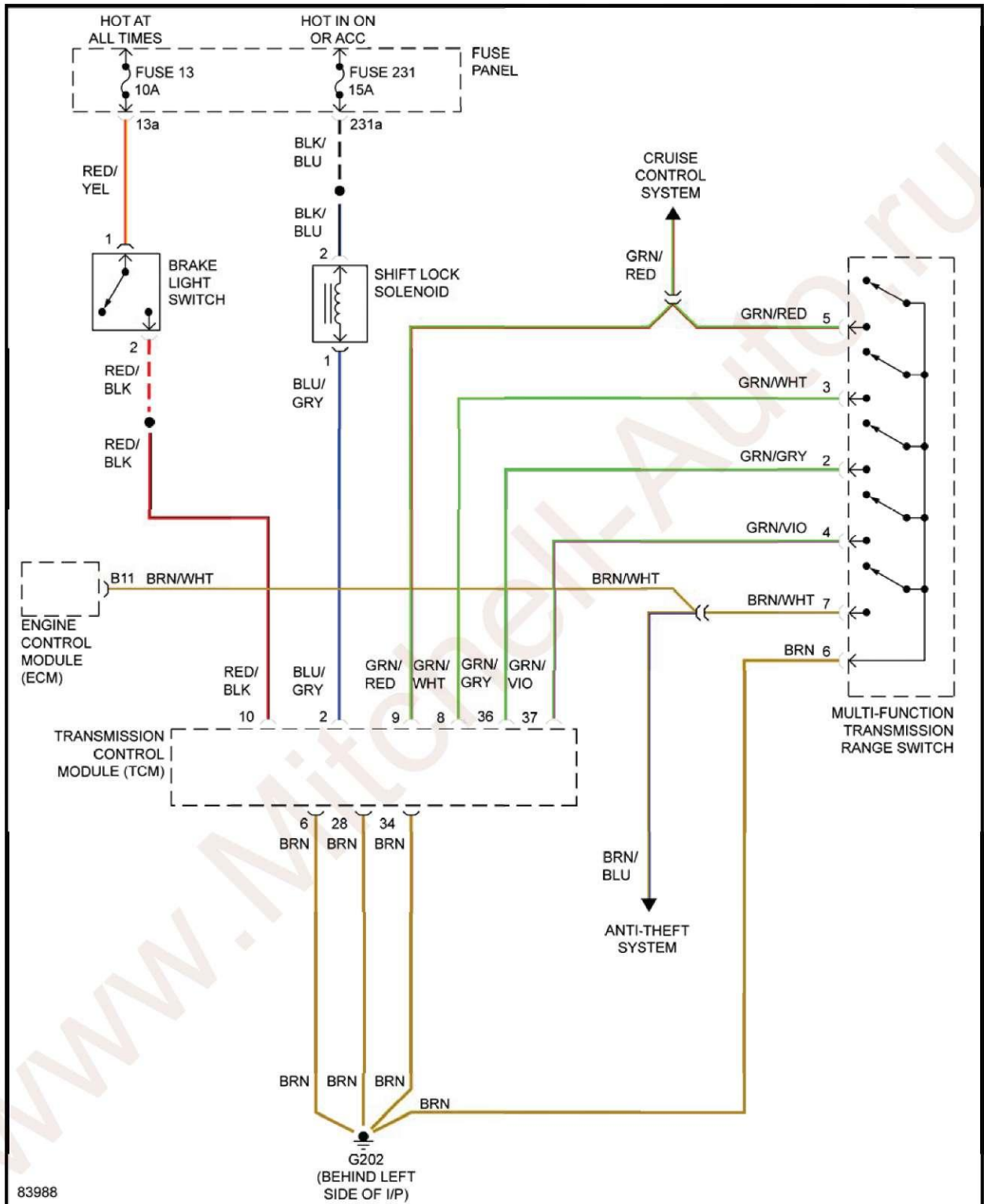
Fig. 33: Shift Interlock Circuit
